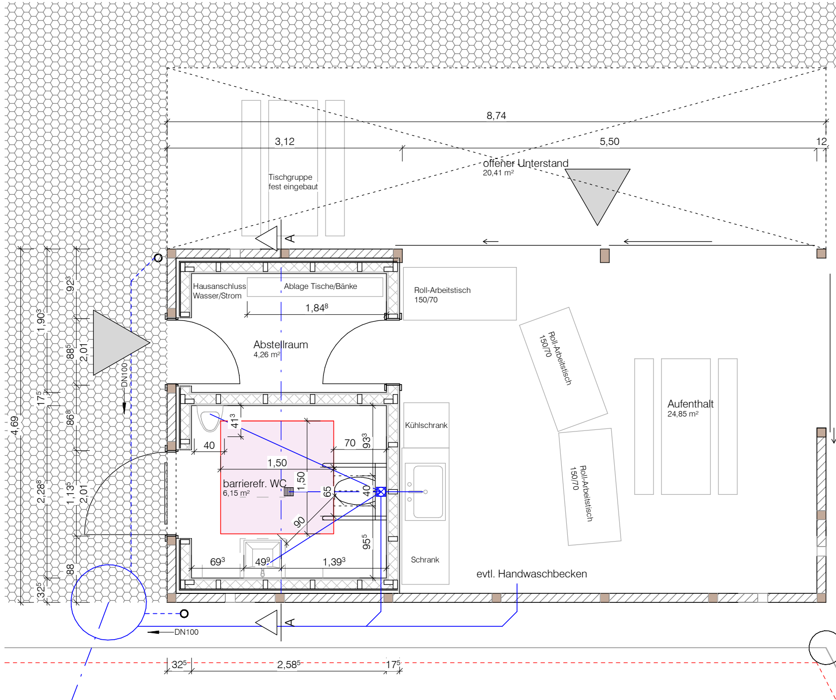
Erdgeschoss 1 : 50
