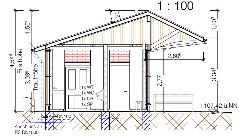
Schnitt A-A 1 : 100
